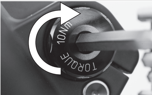
Abbildung 35: Eingesetzte Achse festziehen
