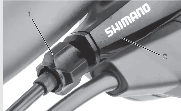
Abbildung 75: Einstellhülse (1) der einzügigen, seilzugbetätigten Gangschaltung mit Schalthebelgehäuse (2), Beispiel
