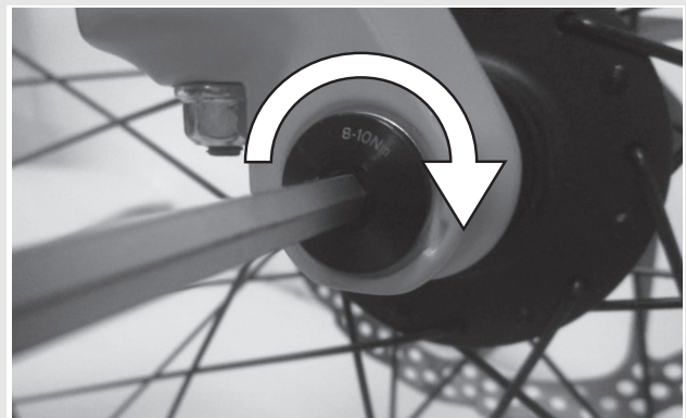
Abbildung 32: Achse anziehen
