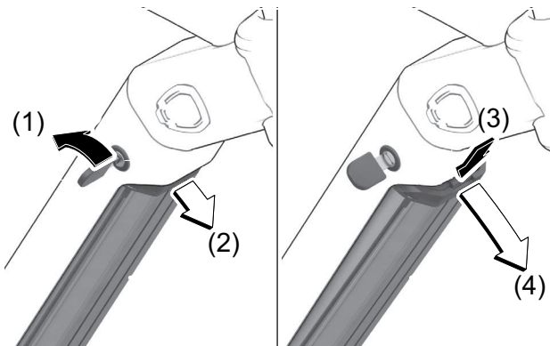
Abbildung 120: Integrierten Akku herausnehmen
