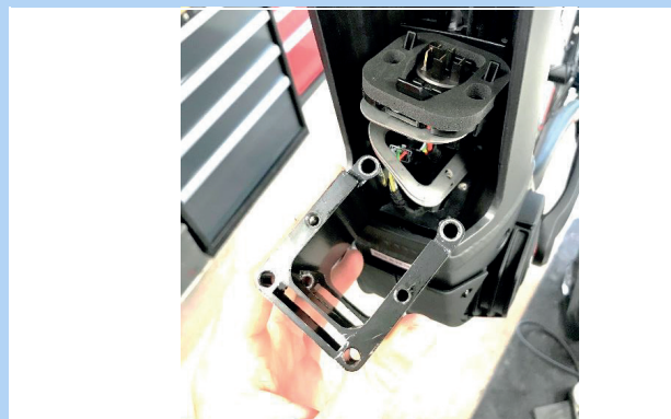
Abbildung 50: PowerTube Adapter herausziehen
