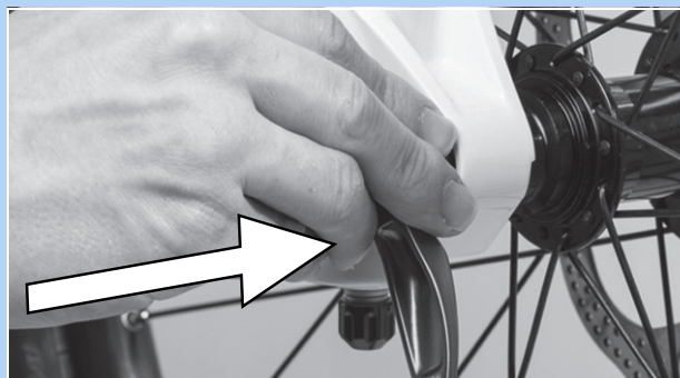
Abbildung 73: Schnellspanner in Pfeilrichtung einschieben
