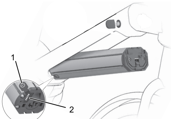
Abbildung 44: Lage Ladezustandsanzeige integrierter Akku
