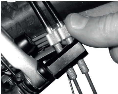
Abbildung 231: ROHLOFF-Naben Versionen mit interner Schaltansteuerung haben die Zugeinsteller am Zuggegenhalter
