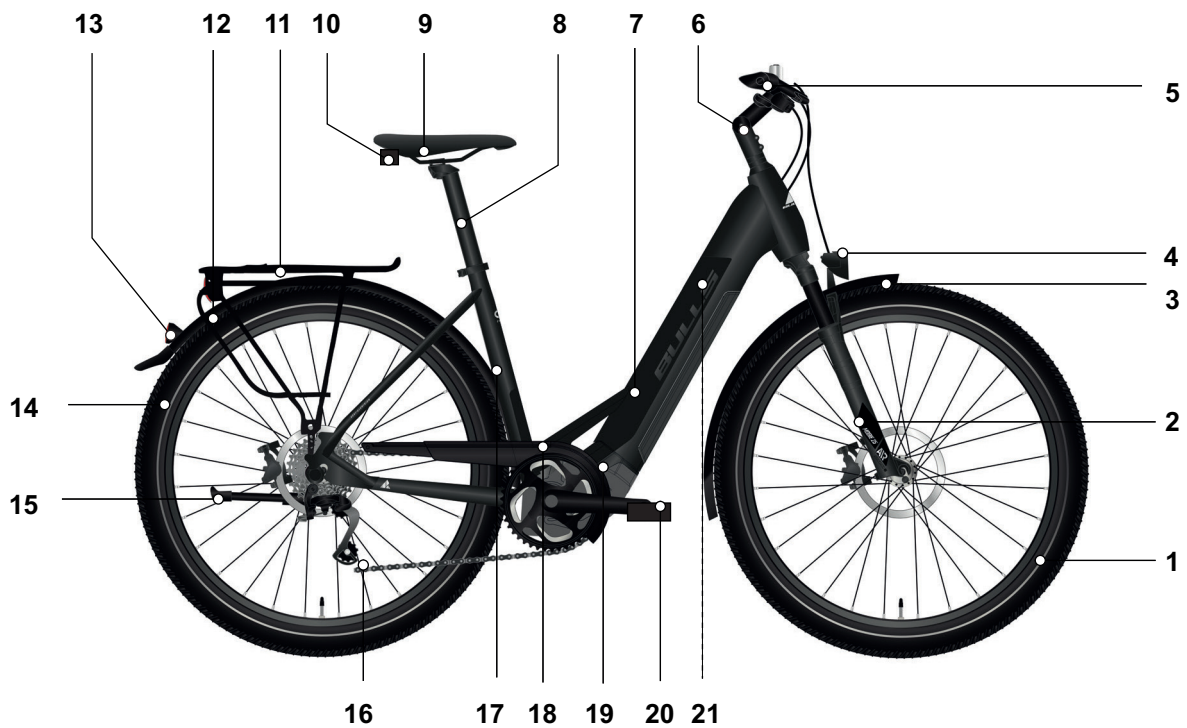
Abbildung 3: Pedelec von rechts, Beispiel BULLS Lacuba EVO 12
