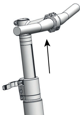
Abbildung 126: Sicherungshebel nach oben ziehen, Beispiel All Up
