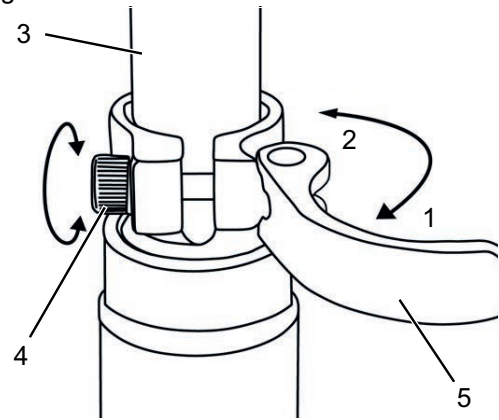
Abbildung 111: Schnellspanner der Sattelstütze öffnen
