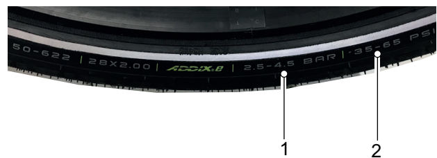
Abbildung 203: Fülldruck in bar (1) und psi (2)
