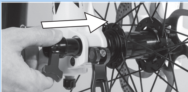
Abbildung 85: Querachse in Pfeilrichtung einschieben
