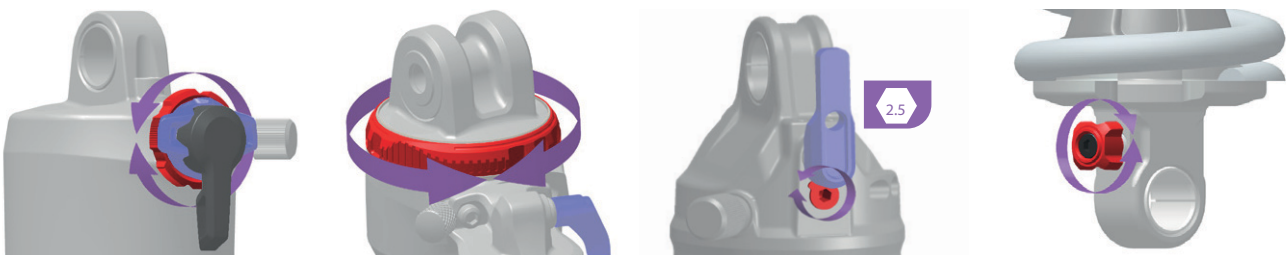
Abbildung 264: Lage und Form des Zugstufen-Einstellers (rot) ist Modellabhängig
