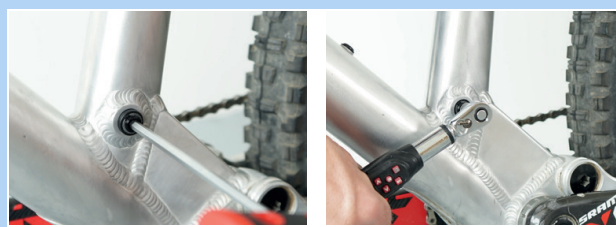
Abbildung 202: Sattelstütze festschrauben
