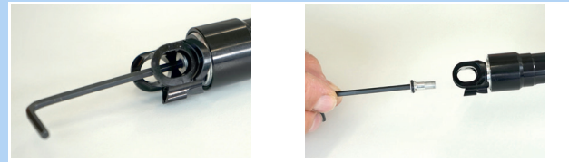
Abbildung 190: Ventilkappe herausdrehen
