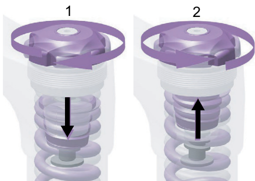
Abbildung 105: Vorspannungseinsteller hinein (1) und heraus (2) drehen.
