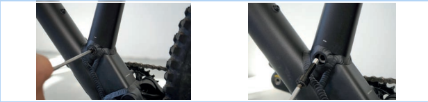
Abbildung 208: Sattelstütze lösen
