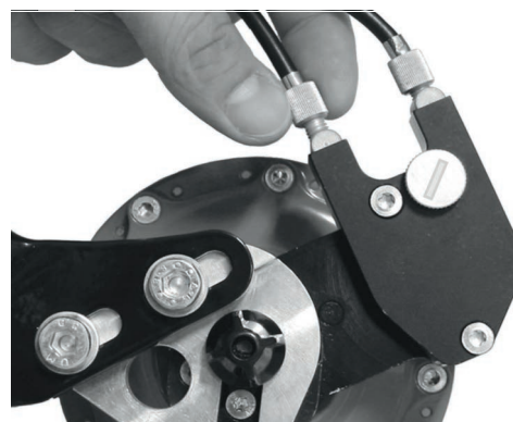
Abbildung 164: ROHLOFF-Naben Versionen mit externer Schaltansteuerung haben die Zugeinsteller an der Seilbox, die sich auf der linken Seite befindet
