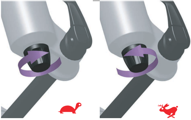
Abbildung 118: ROCKSHOX Zugstufe einstellen
