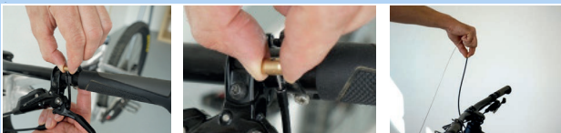
Abbildung 209: Fernbedienung lösen
