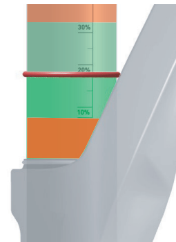
Abbildung 112: Vorgeschriebener SAG Bereich (grün) und verbotener SAG Bereich (rot)
