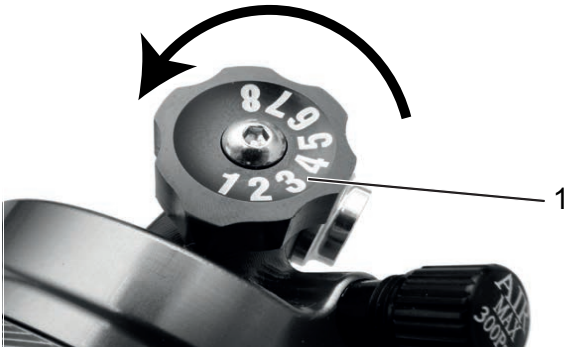
Abbildung 122: Suntour-Druckstufeneinsteller (1) am Hinterbau-Dämpfer
