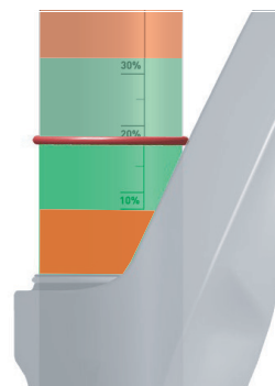
Abbildung 102: Vorgeschriebener SAG Bereich (grün) und verbotener SAG Bereich (rot)
