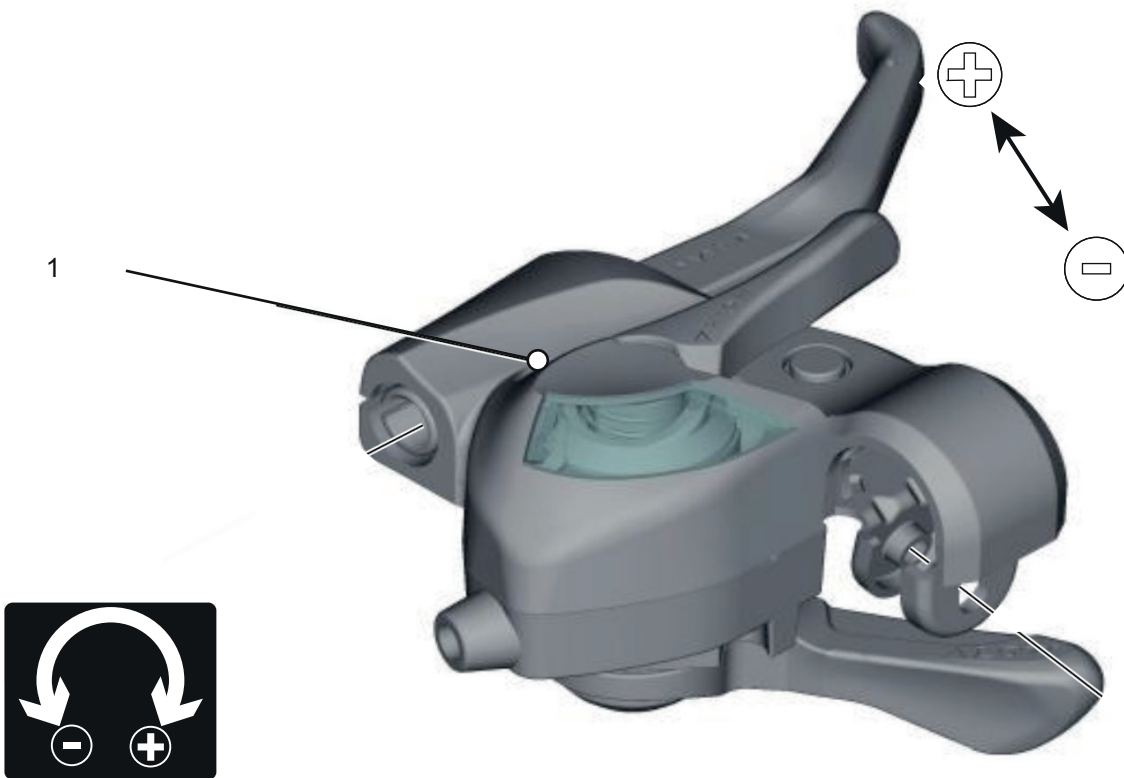
Abbildung 97: Lage Stellschraube (1)
