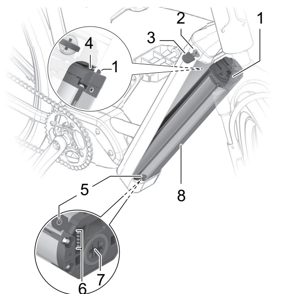
Abbildung 40: Detail PowerTube 750
