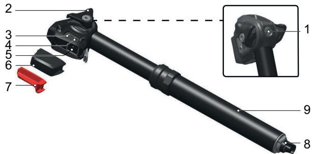
Abbildung 33: Aufbau ROCKSHOX Reverb AXS Sattelstütze
