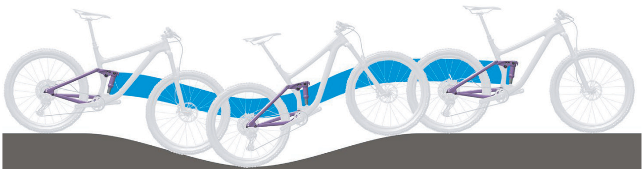
Abbildung 22: Optimales Fahrverhalten des Hinterbau-Dämpfers im hügeligen Gelände
