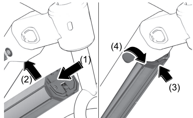
Abbildung 110: Integrierten Akku einsetzen
