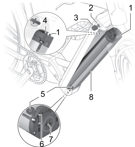
Abbildung 31: Detail PowerTube 750
