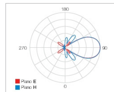
Diagrama de radiación
