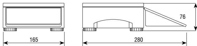
Dimensiones (mm)
