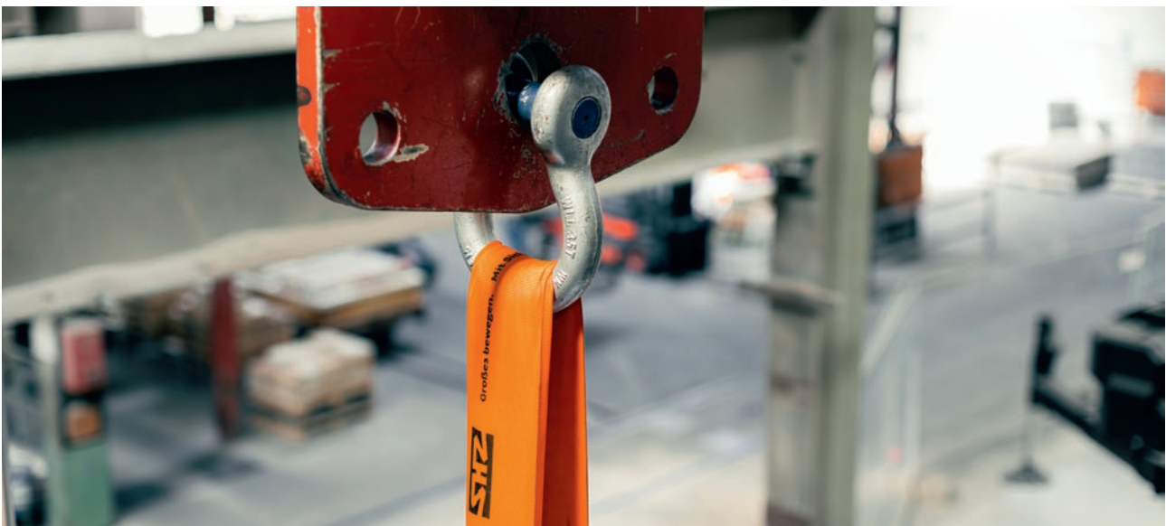
Kombination Schäkel mit Schwerlastrundschnge
