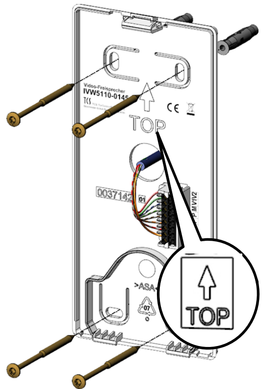
Abb. 3: Montageschale montieren
