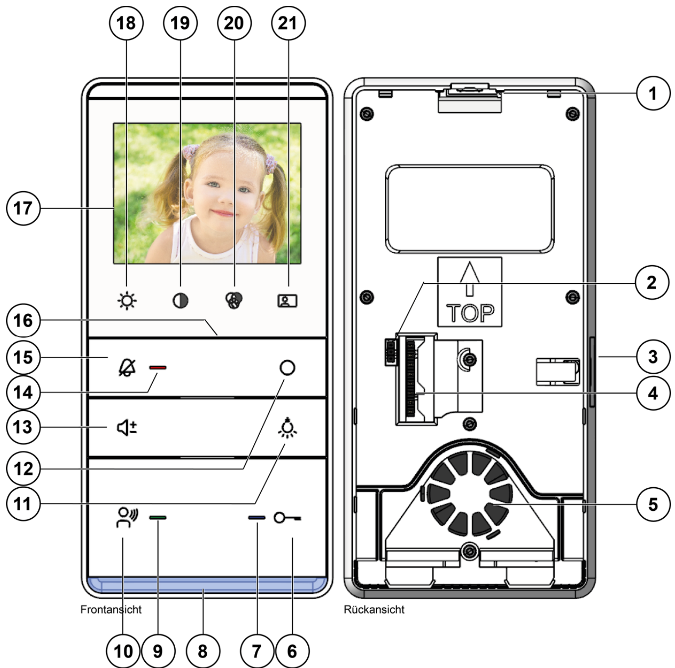
Abb. 1: Geräteübersicht
