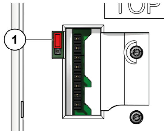
Abb. 6: Abschlusswiderstand aktiviert
