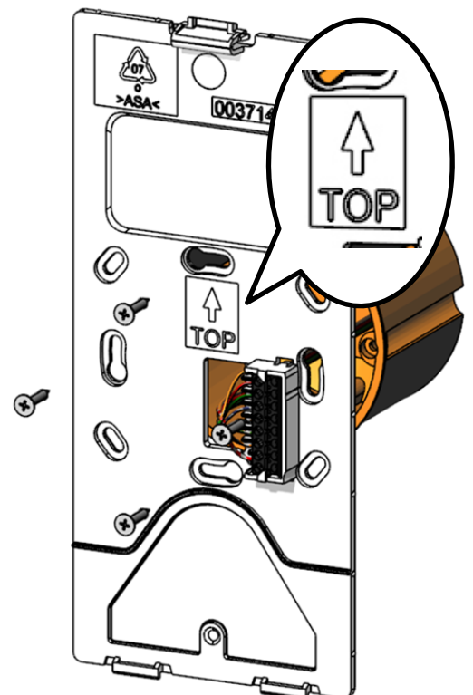
Abb. 4: Montageplatte montieren
